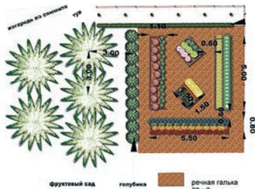
Декоративний огоро́д Масштаб 1:200
